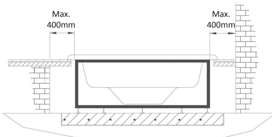
Schema minimumafstand rondom de Spa.
