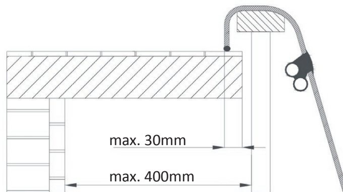
Detalle Sellado Pestaña
