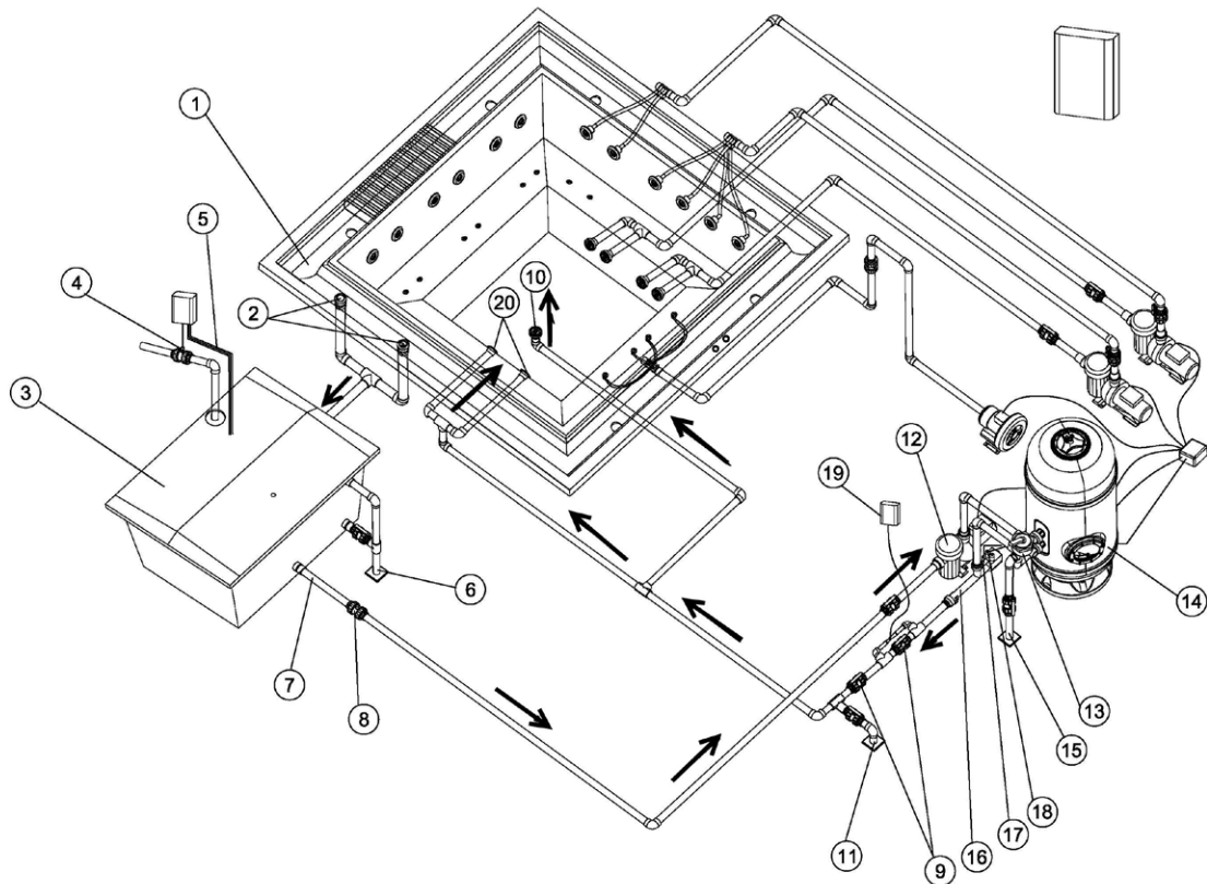
Esquema recirculación Spa con Desbordante. Opción B.
