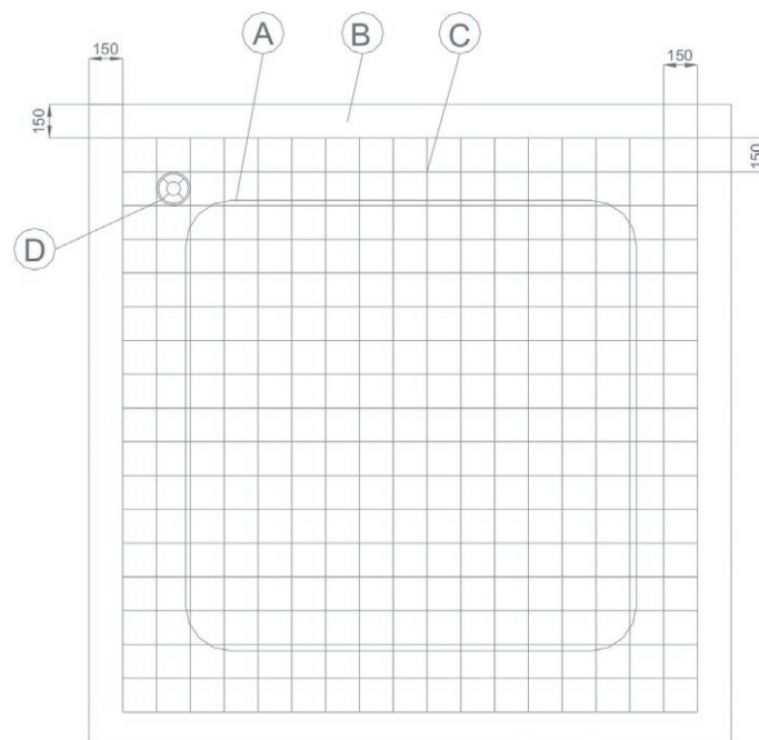
Esquema Cimentación.
