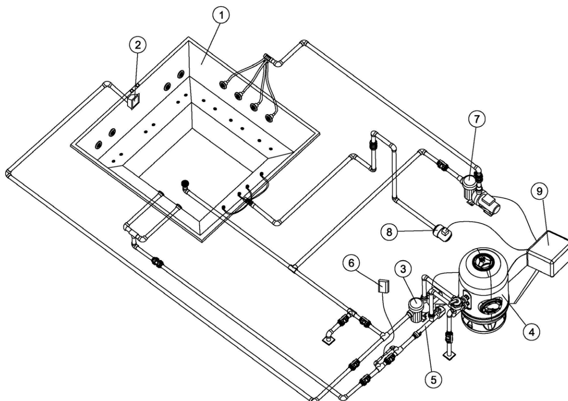
Esquema geral Spa com Skimmer.
