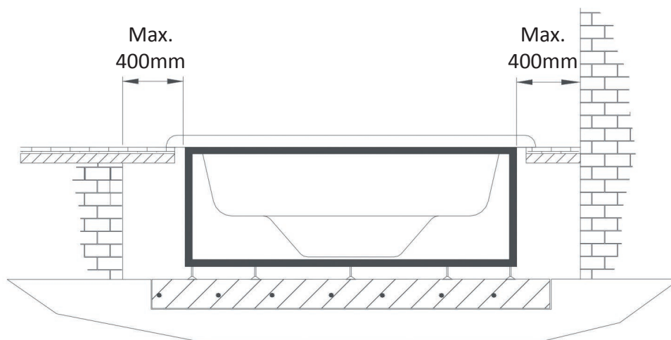
Schéma Distance minimum autour du Spa.
