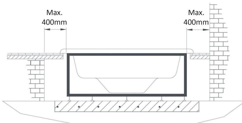
Esquema Distância mínima à volta do Spa.
