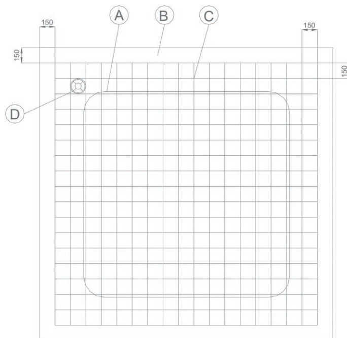
Schema basamento.
