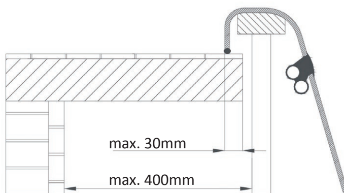
Detalhe do lábio de vedação
