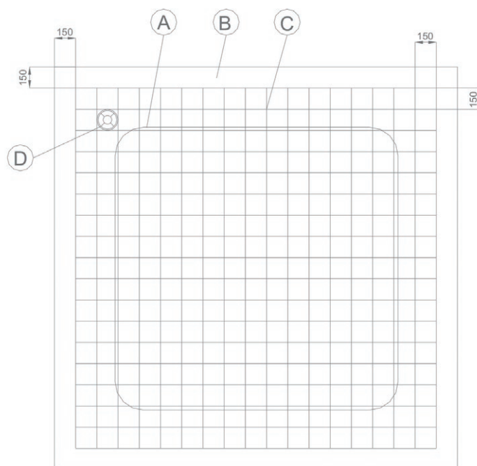
Schéma Cimentation
