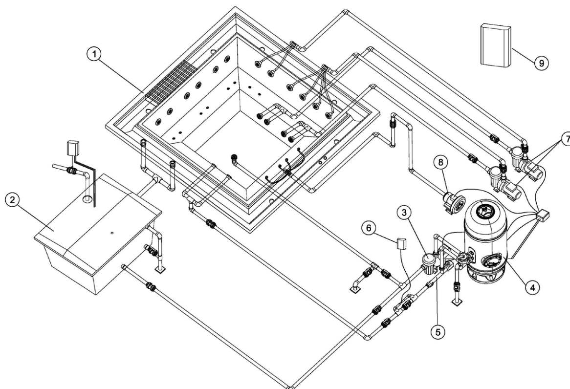
Overzichtsschema Spa met Afvloeiing.
