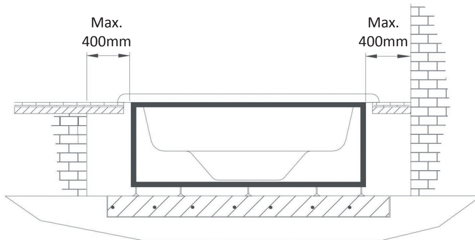
Esquema Distancia mínima alrededor del Spa
