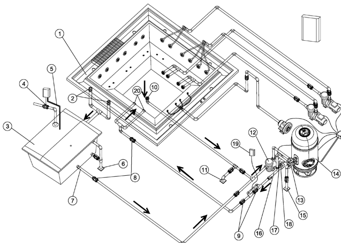
Esquema recirculación Spa con Desbordante. Opción A.
