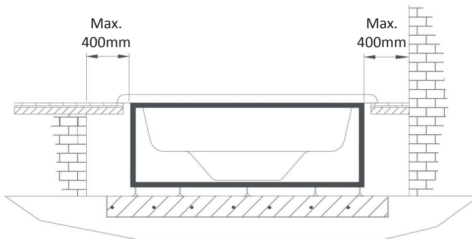
Schaubild Mindestabstand um das Spa.
