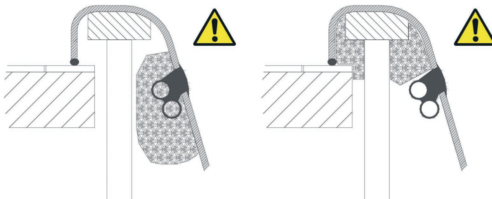
Detalhe Não encher.
