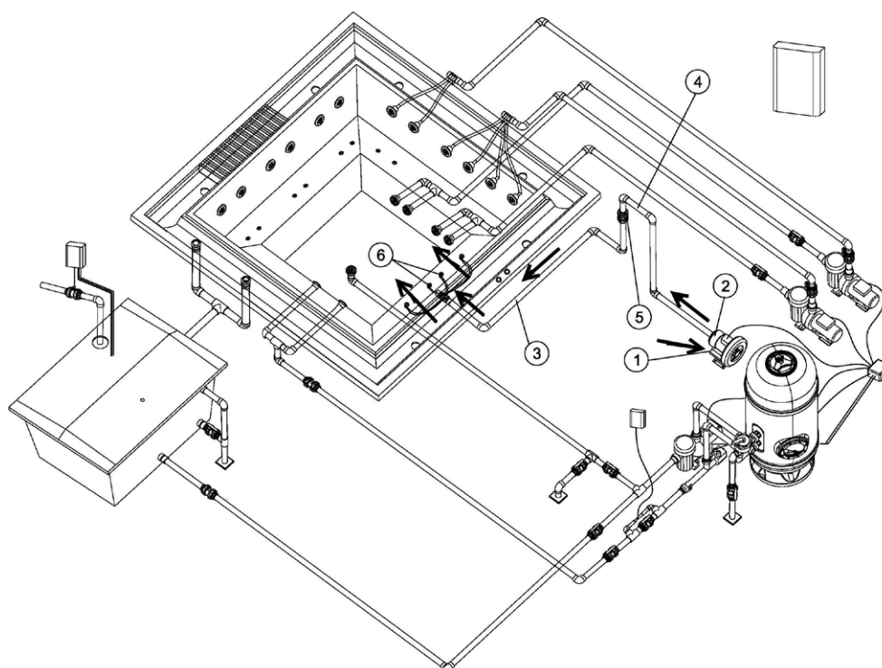
Schema Luchtmassage Spa.
