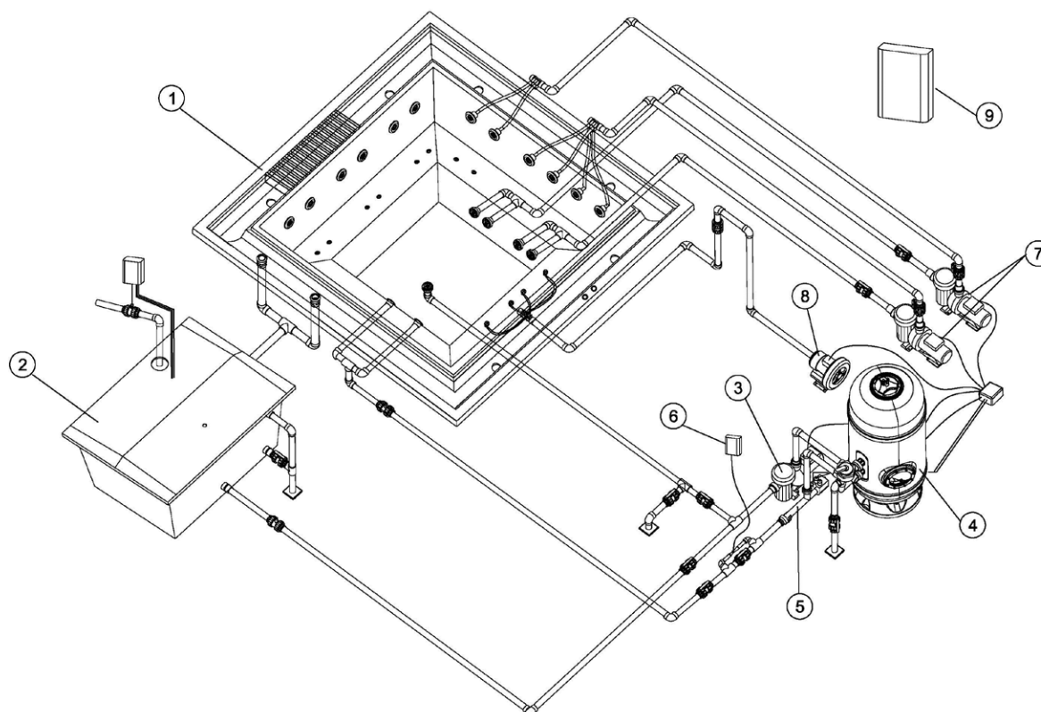
Schema generale Spa a bordo sfioratore.
