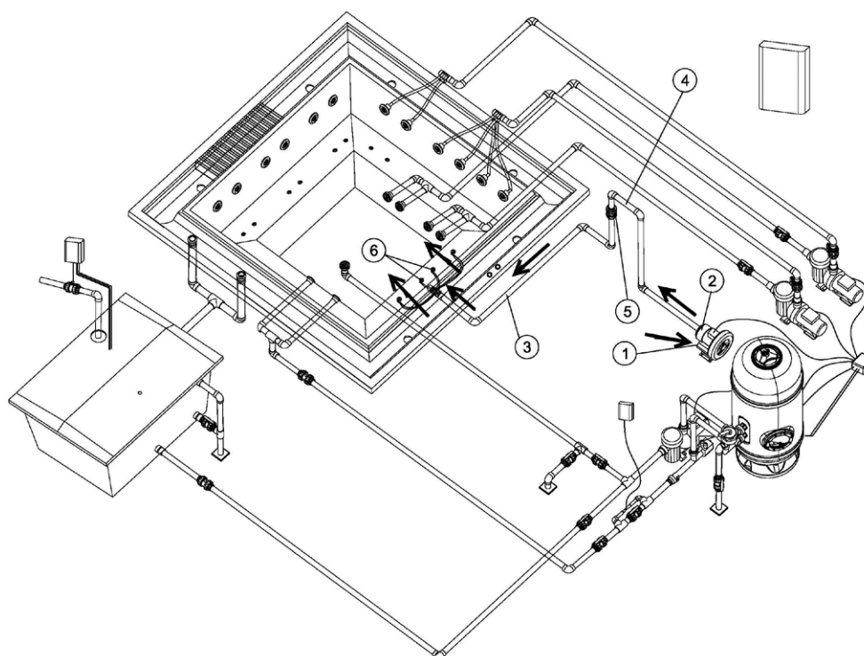
Schéma Massage à air Spa.
