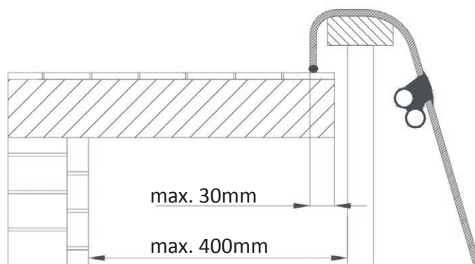
Détail Scellement rebord.
