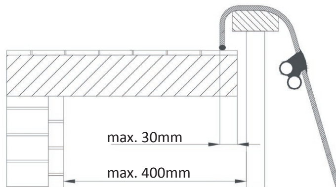
Einzeldarstellung der Versiegelung vom Flansch.
