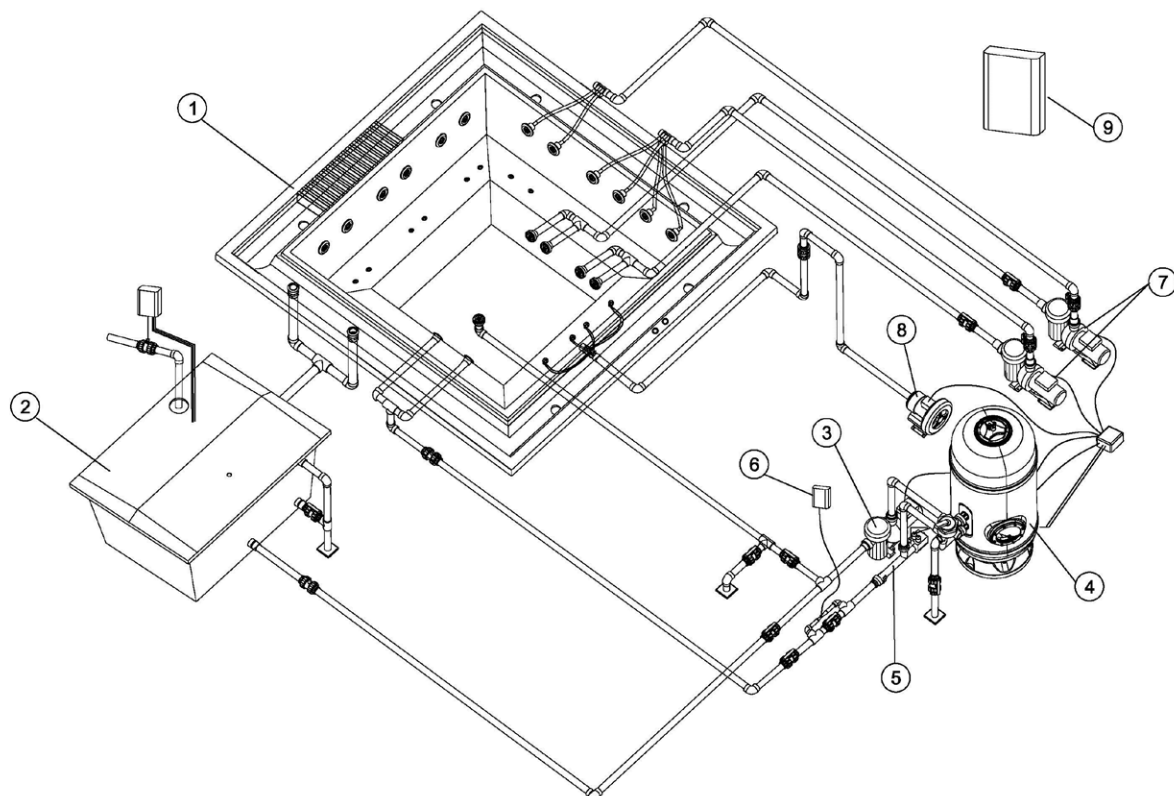
Schéma général d'un Spa à débordement.
