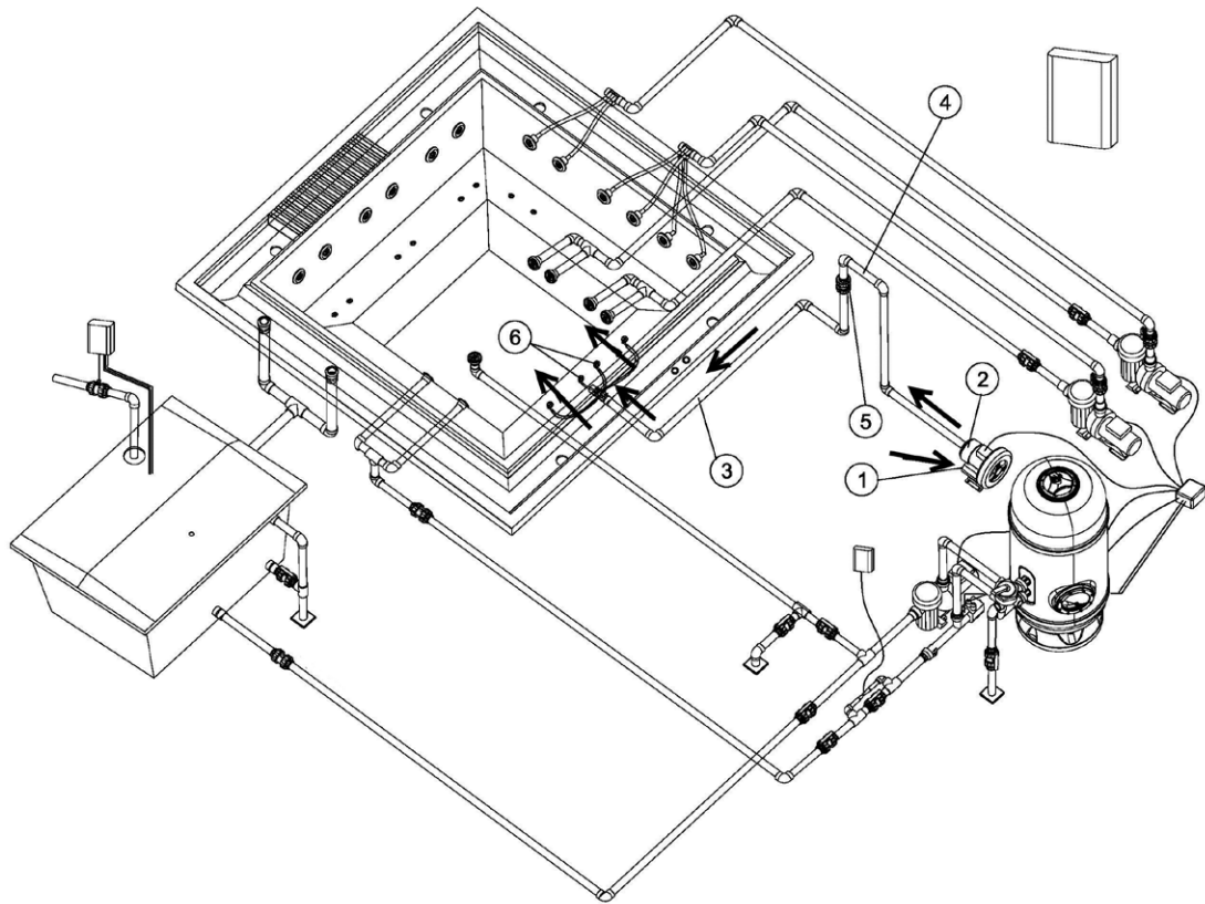
Schema Luftmassage Spa
