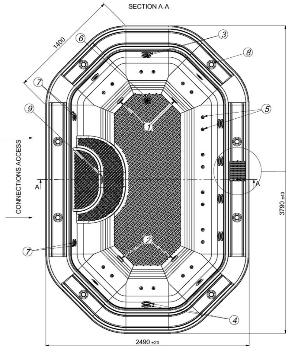
SECTION A-A
